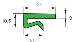
Perfil P 25 - Verde P 25 Profile - Green Profil P 25 - Vert
