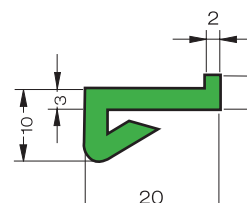
Perfil P 20 - Verde P 20 Profile - Green Profil P 20 - Vert
